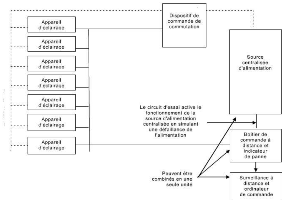
Figure A.4 – Connexion directe entre appareils d'éclairage et le boîtier de commande à distance
