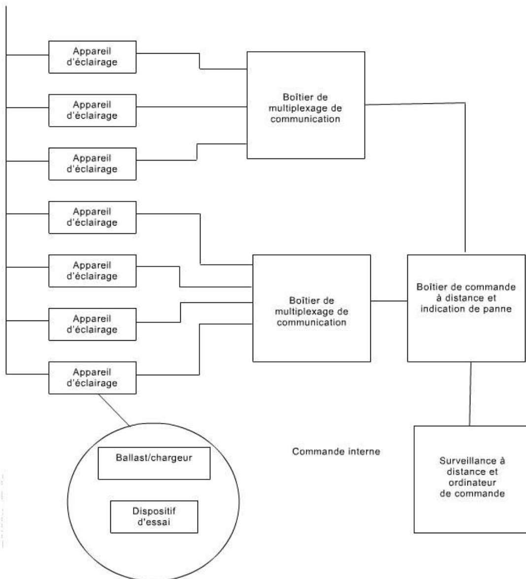
Figure A.3 – Variante du système où la liaison des appareils d'éclairage vers le dispositif de signalisation et de contrôle à distance se fait via un boîtier de multiplexage
