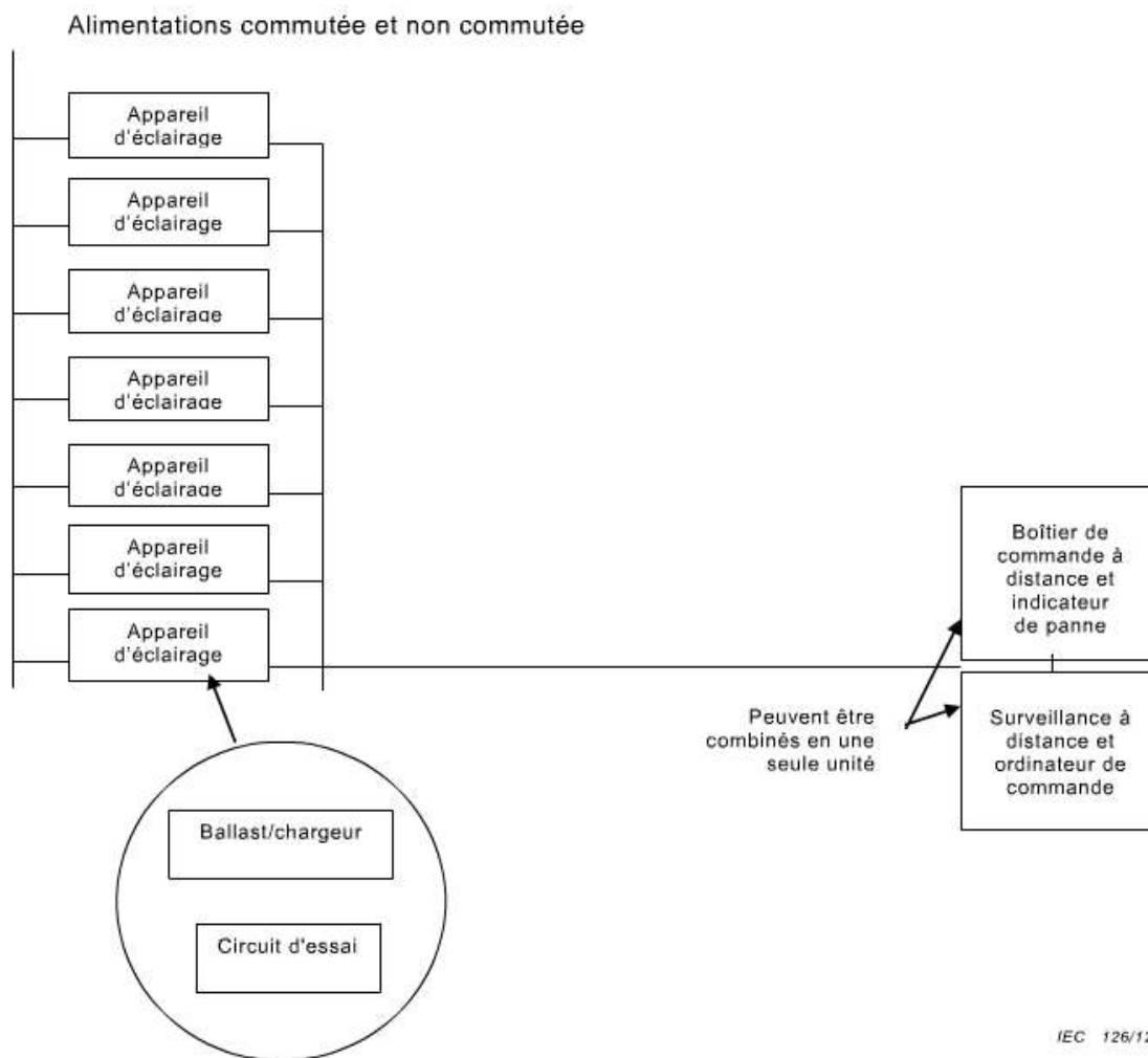
Figure A.2 – Connexion directe entre appareils d'éclairage et boîtier de commande à distance
